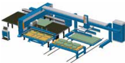
Uusi Prima Power PG 1530, levytyökeskus varustettuna LST-robotilla on aikaisemmin investoidun sisarkone.
